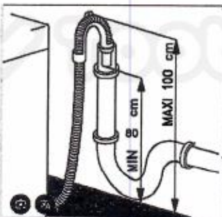
Правильный изгиб шланга
